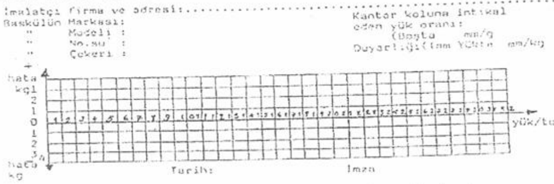
Şekil: 2- Kantar kolu taksimat aralıkları hata çizelgesi
